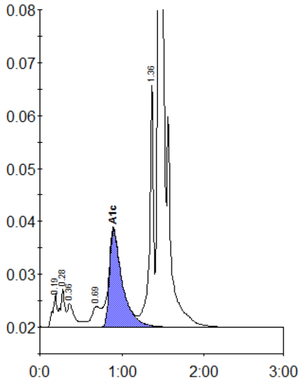
Peak table - ID: 10614860
